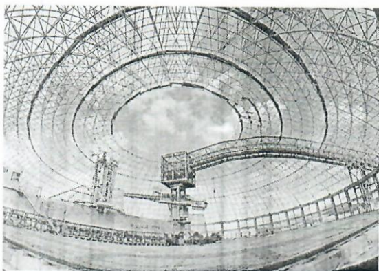
Hình ảnh 7: Giàn không gian CKDA xuất khẩu sang Namibia-Châu Phi
