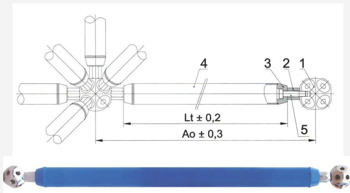
1. Nút cầu 2. Ống lồng 3. Đầu côn 4. Thanh giàn 5. Bu lông cường độ cao
